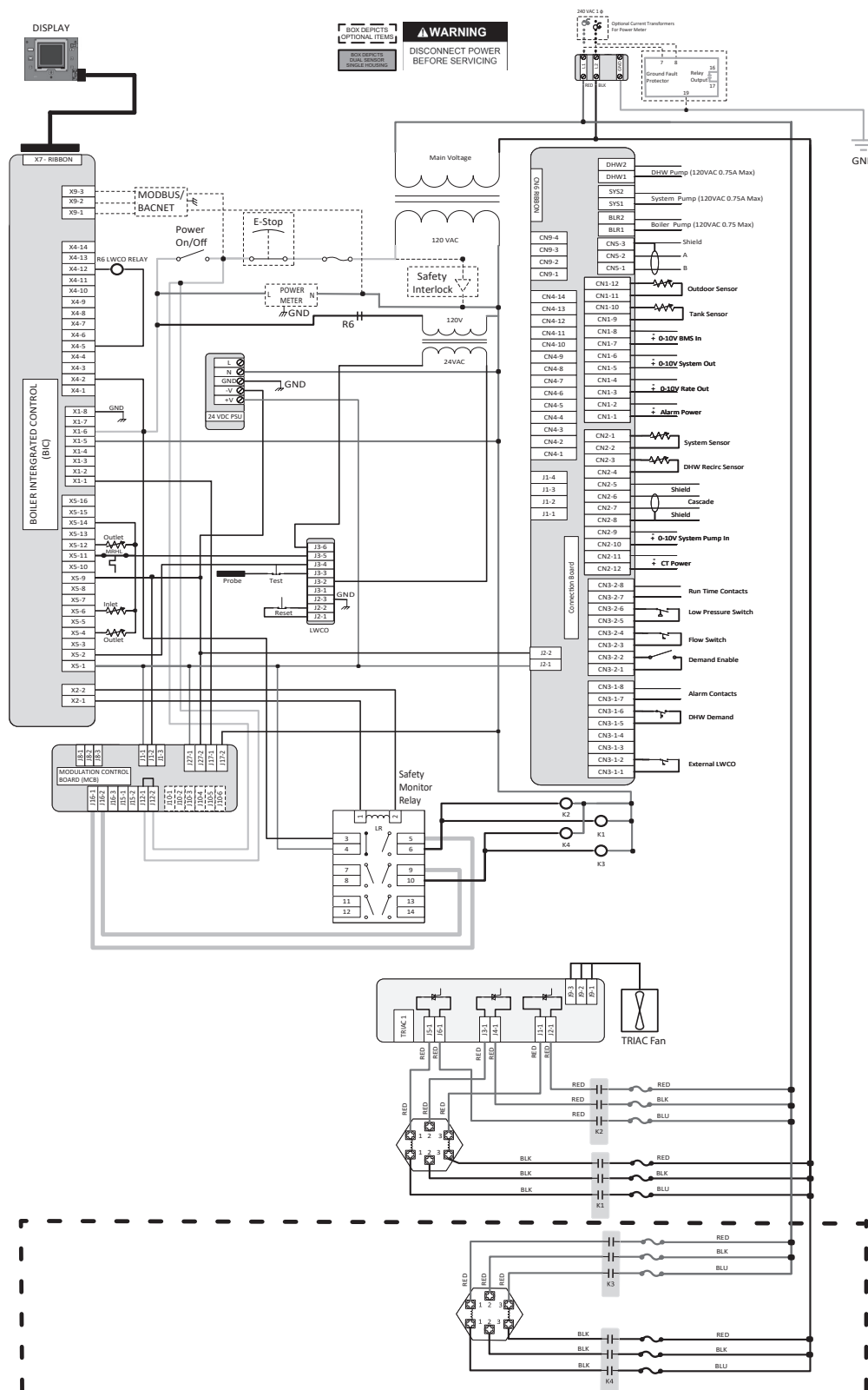
Figure 8-8 Schéma électrique - 240V, 1 Phase (A)
